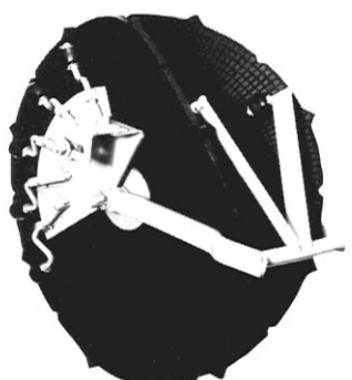
Gummiskiveplantejul for planting af såvel barrodsplanter som pottede planter
