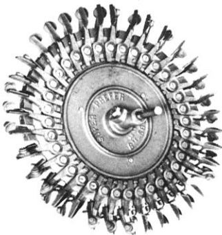
Plantehjul med fjederpåvirkede gribere for plantning af barrodsplanter
