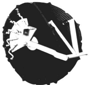
Gummiskiveplantehjul for planting af såvel barrodsplanter som pottede planter
